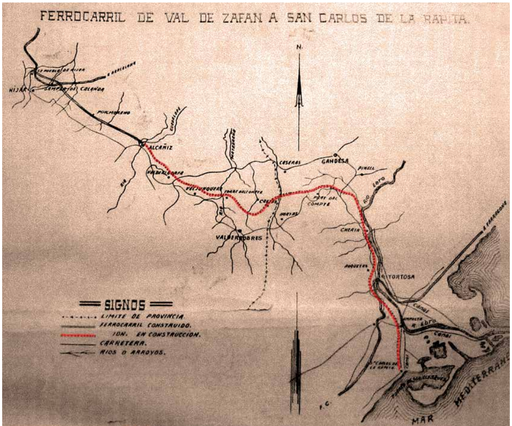
Plànol del traçat de la via de Val de Zafán, des de Puebla de Híjar fins Sant Carles de la Ràpita. El tram en roig correspon al que va des d'Alcañiz fins la Ràpita.
